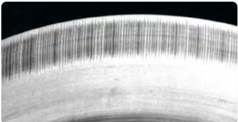
Канавки, характеризующие электрическую эрозию в подшипнике
