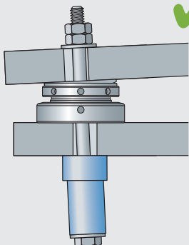
Прямой болт
